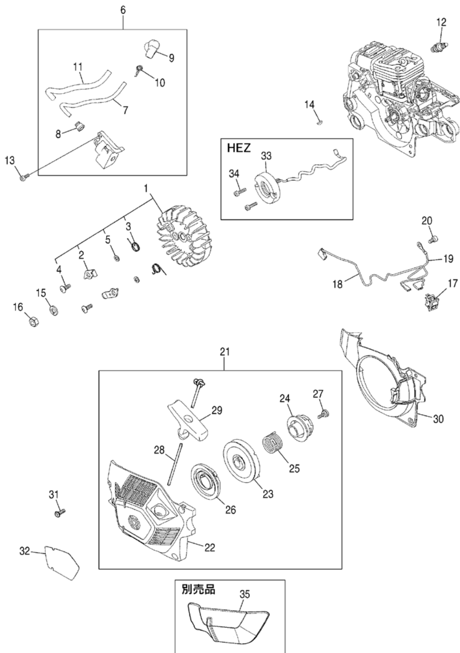
図3 電装・スタート
