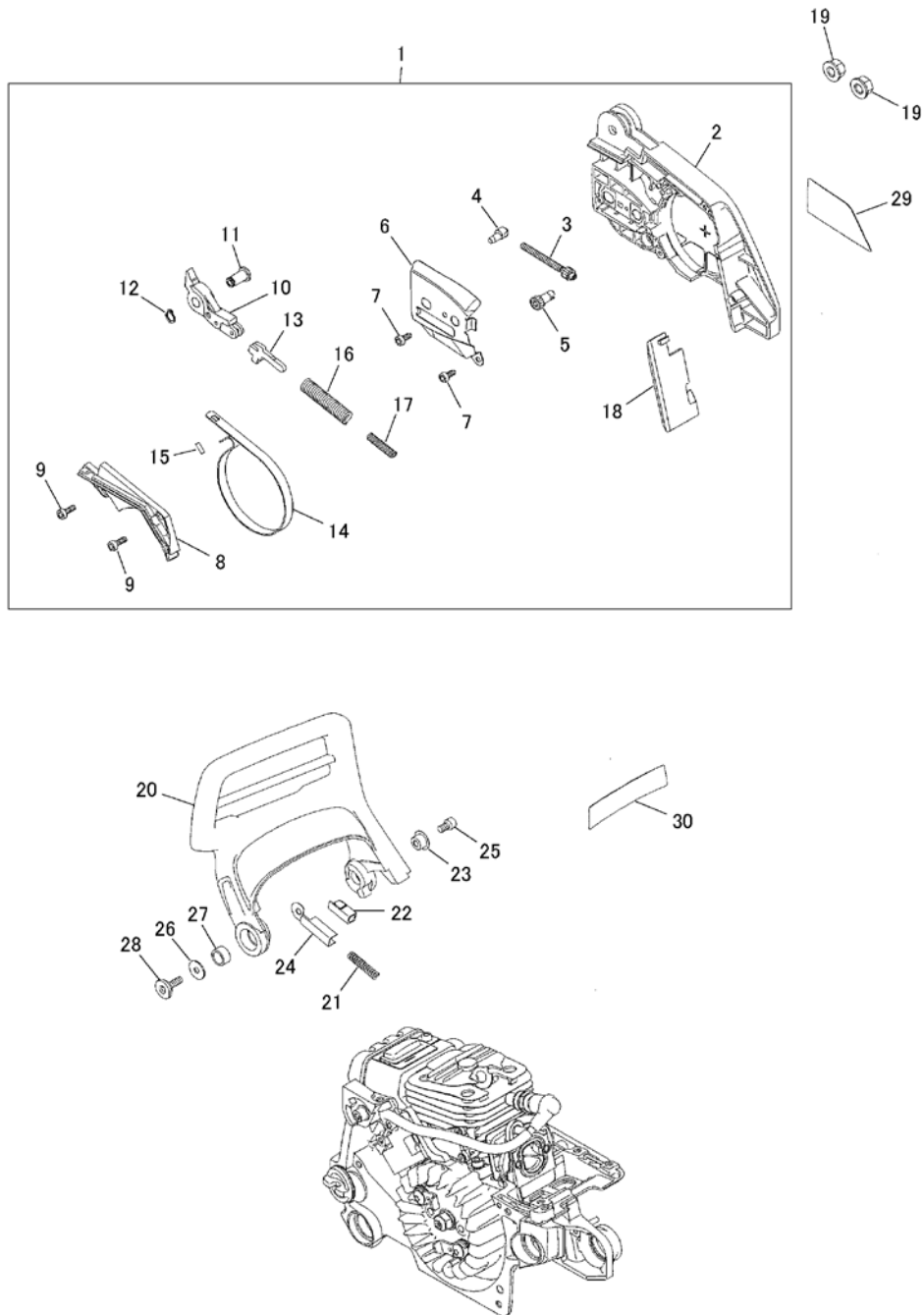
図6 クラッチカバー・フロントガード
