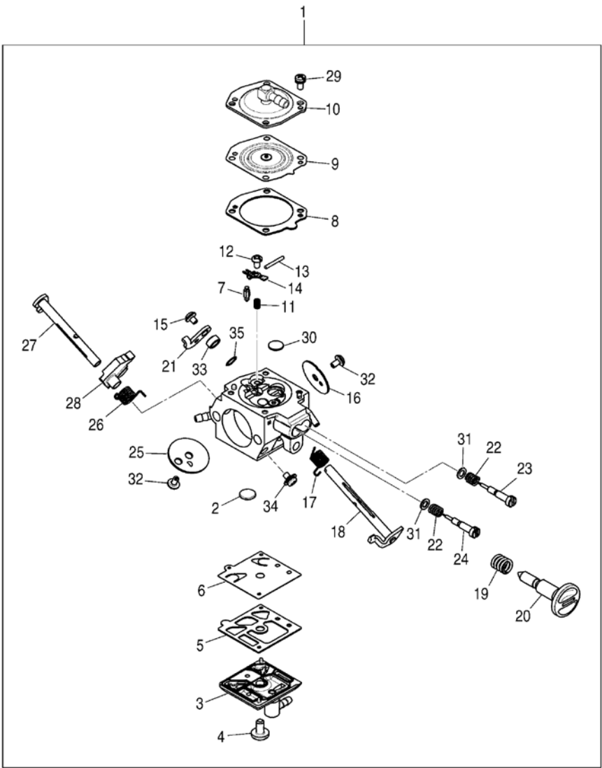
図8 キャブレタ
