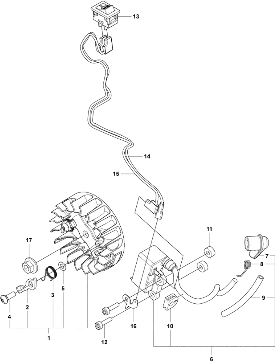
図8 電装
