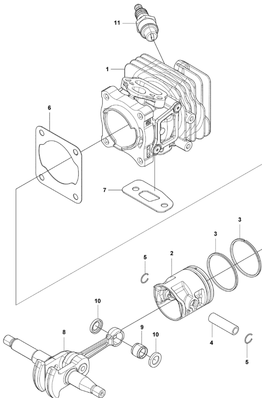
図1 シリンダ・ピストン・クランクシャフト
