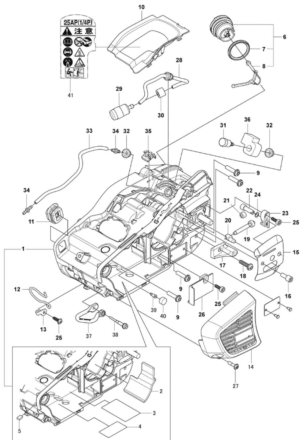
図6 ハウジング
