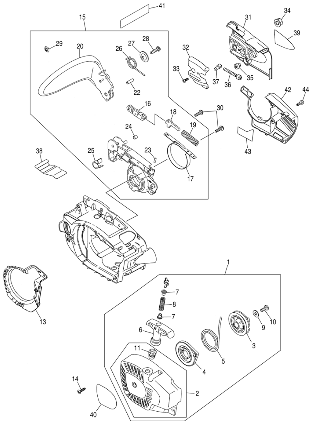
図4 スタータ・ブレーキ・チェンカバー
