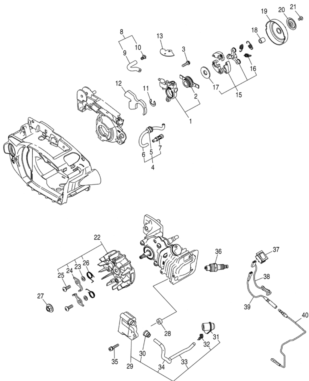
図2 オイルポンプ・クラッチ・電装
