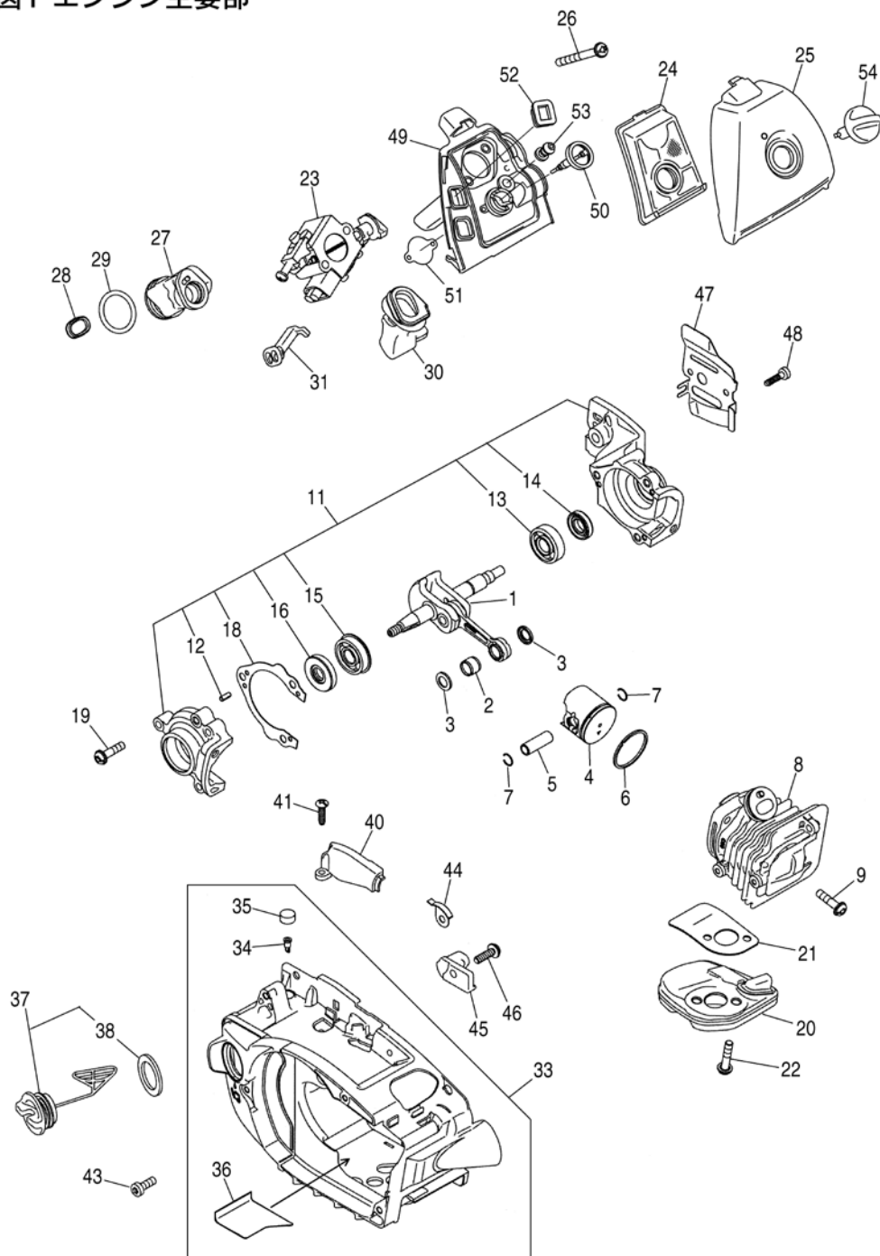
図1 エンジン主要部
