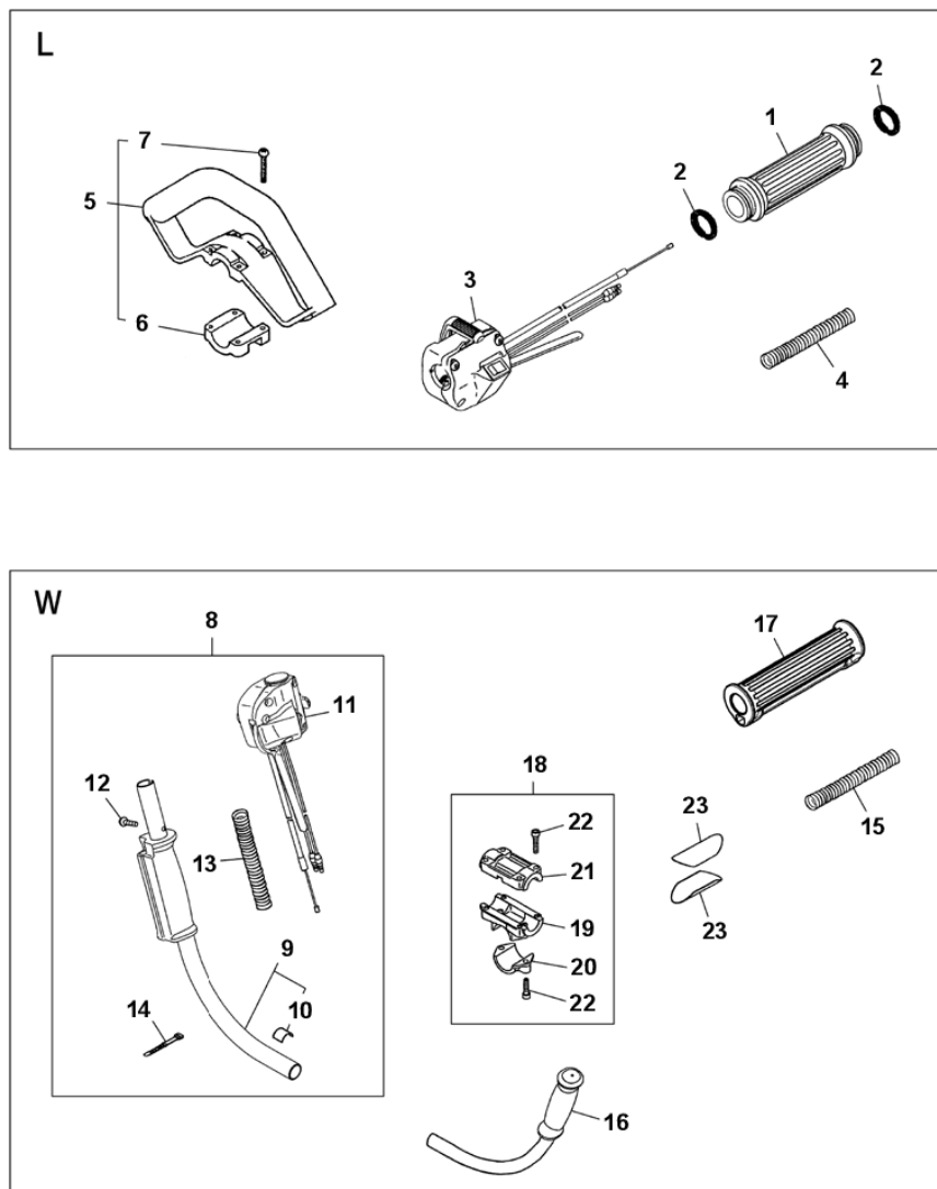
図5 ハンドル回り(STレバー)
