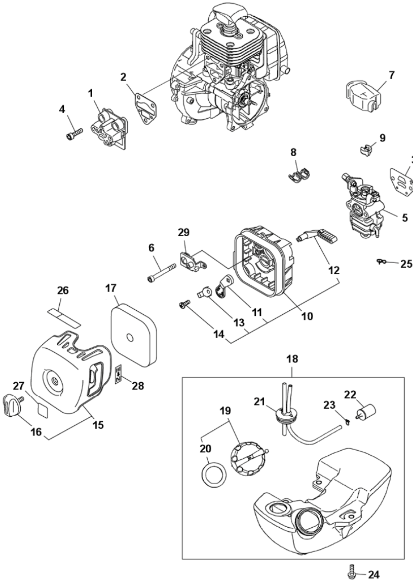
図2 燃料供給系
