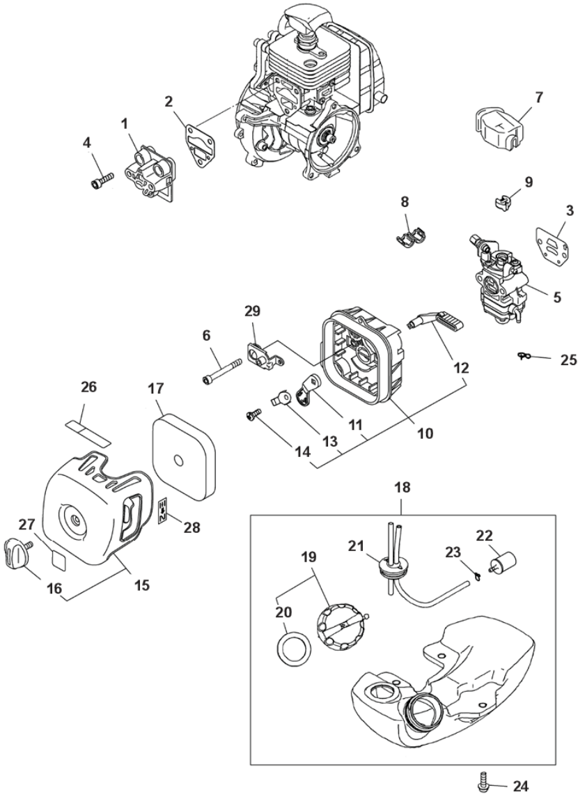
図2 燃料供給系
