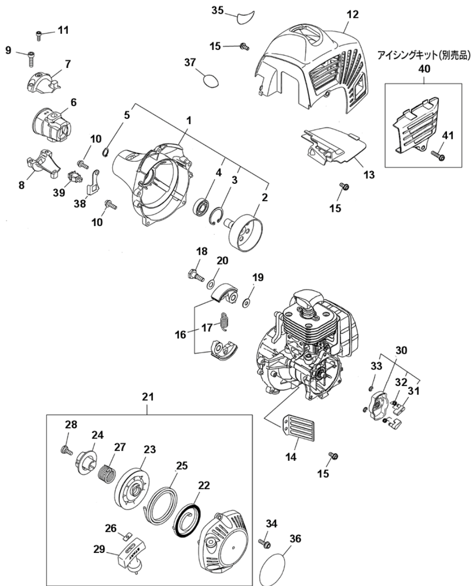
図3 外装・クラッチ・スタータ
