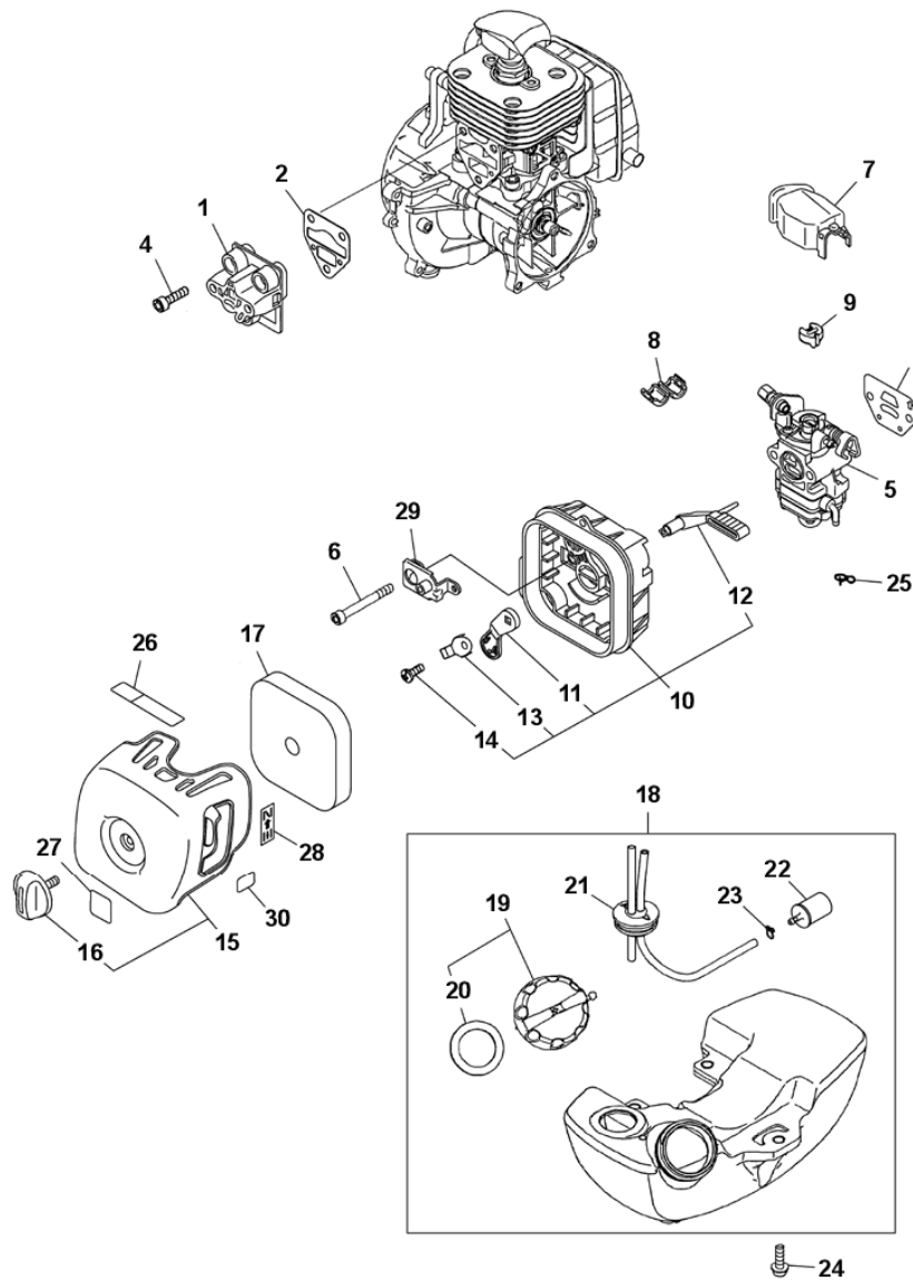
図2 燃料供給系
