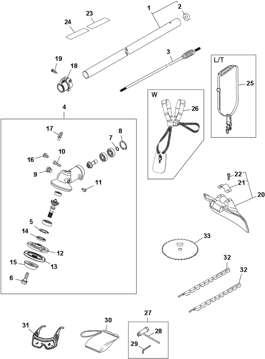
図4 操作桿・付属品
