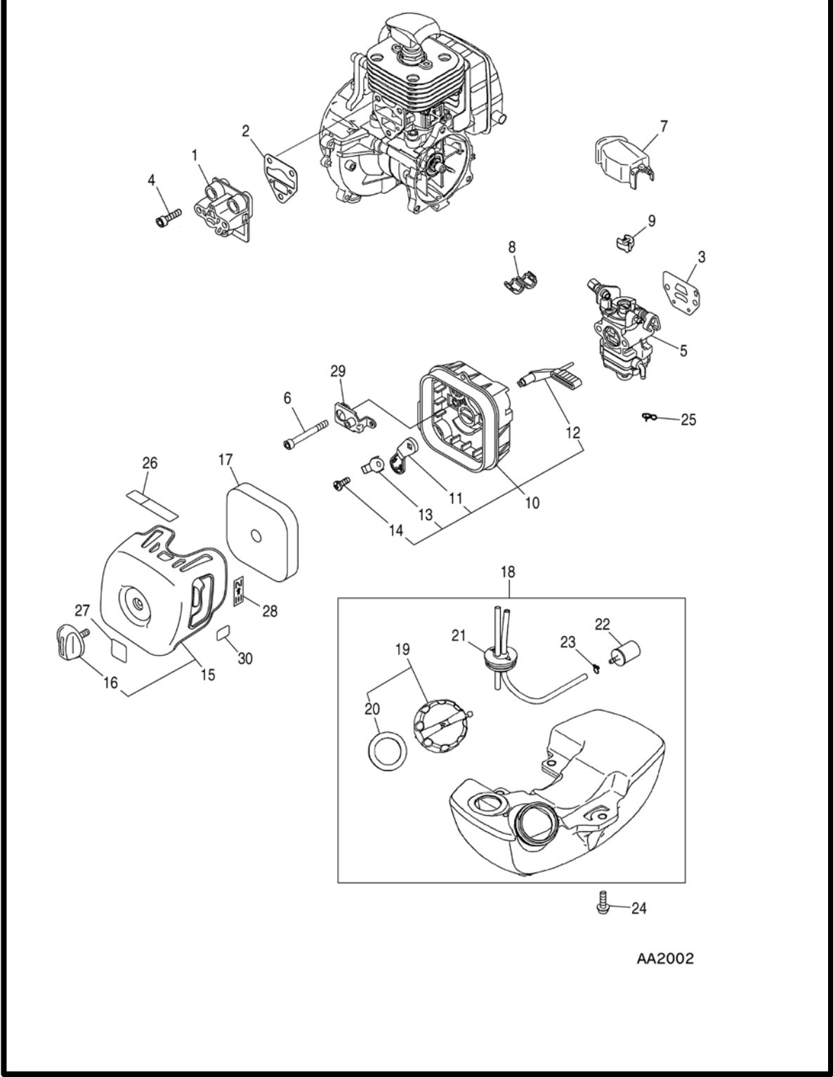
図2 燃料供給系
