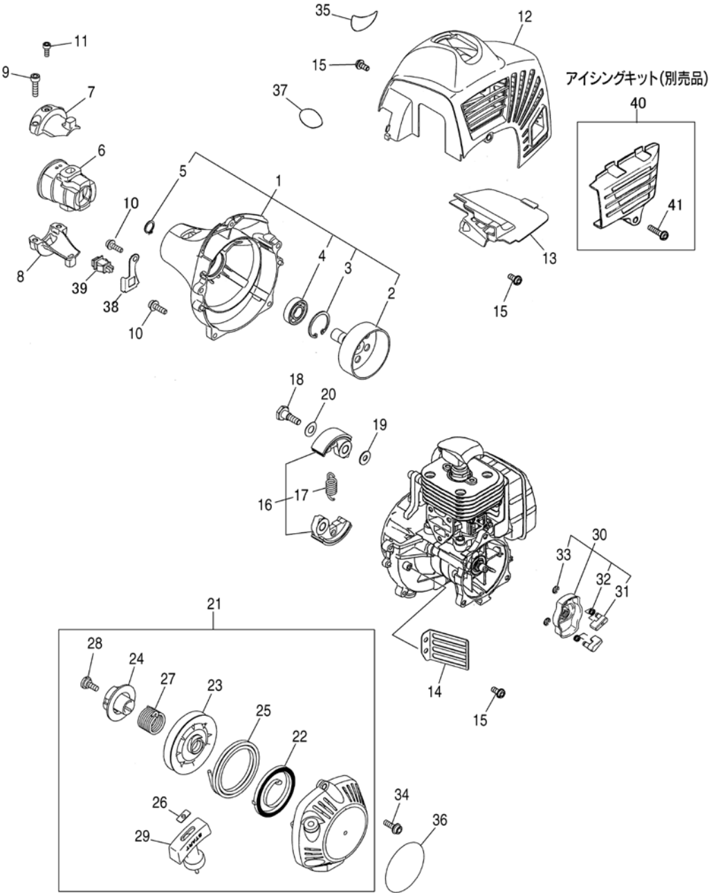
図3 外装・クラッチ・スタータ
