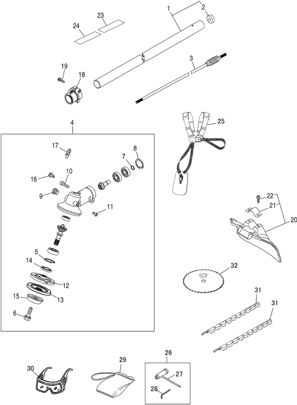
図4 操作桿・付属品
