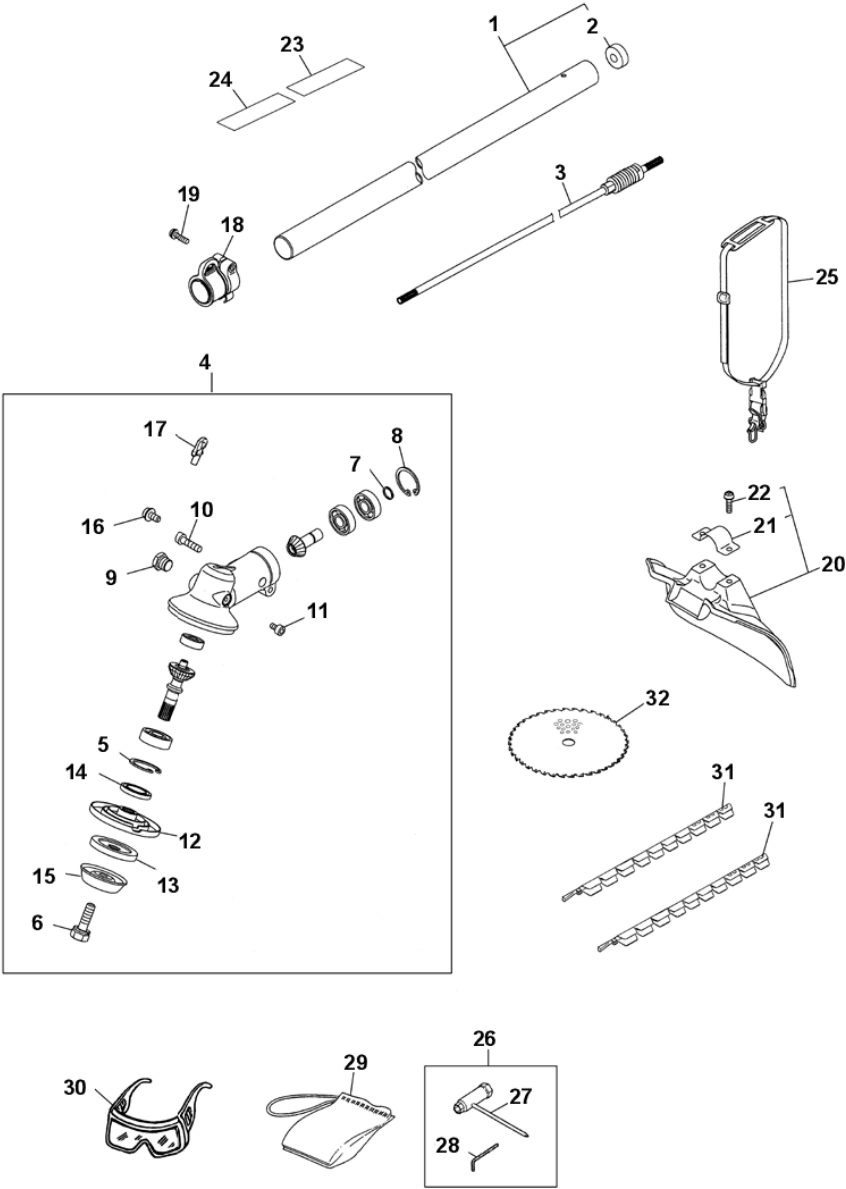
図4 操作桿・付属品
