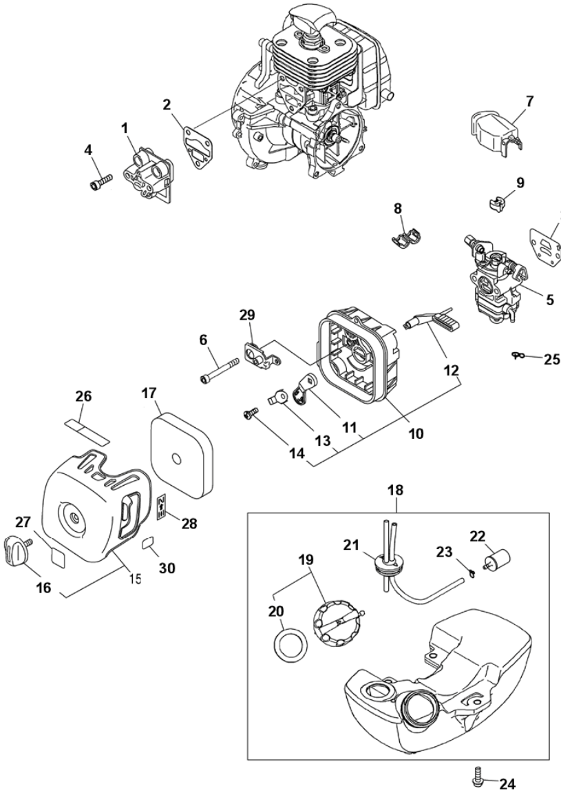
図2 燃料供給系
