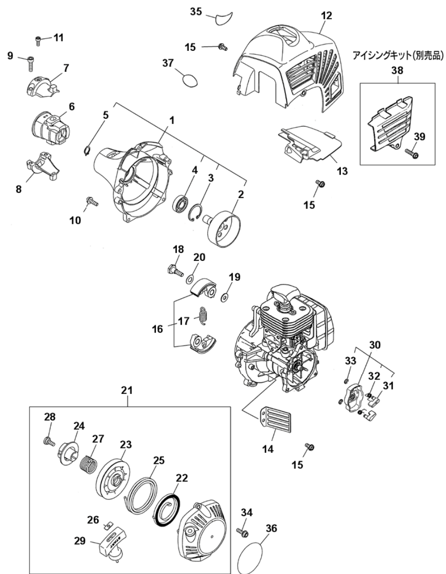
図3 外装・クラッチ・スタータ
