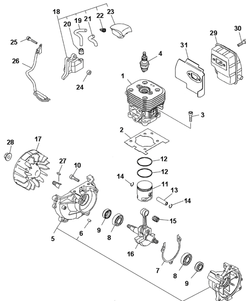
図1 エンジンブロック・電装・マフラ
