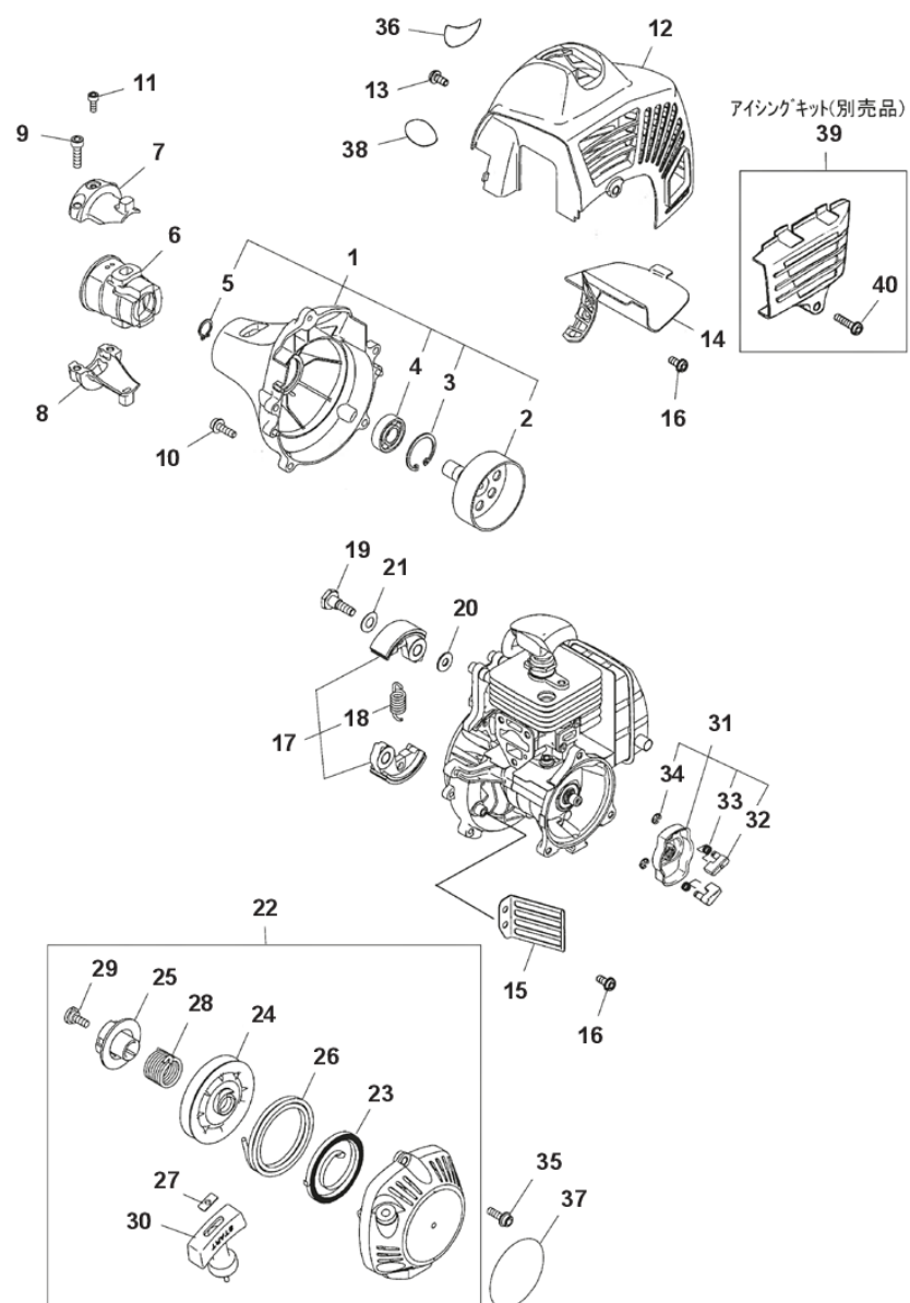
図3 外装・クラッチ・スタータ
