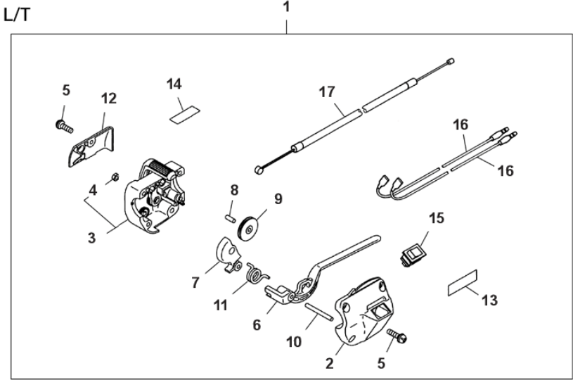
図6 スロットルレバー
