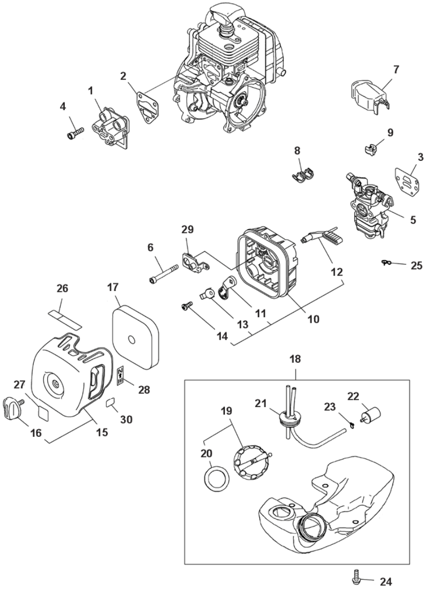
図2 燃料供給系
