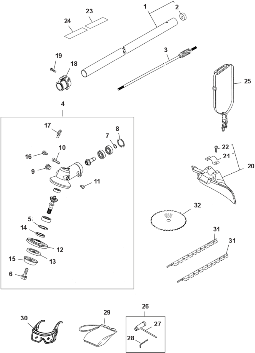
図4 操作桿・付属品
