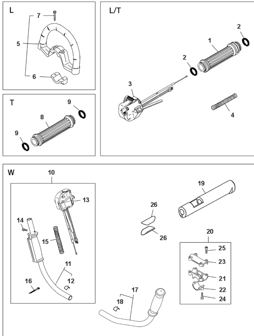
図5 ハンドル回り
