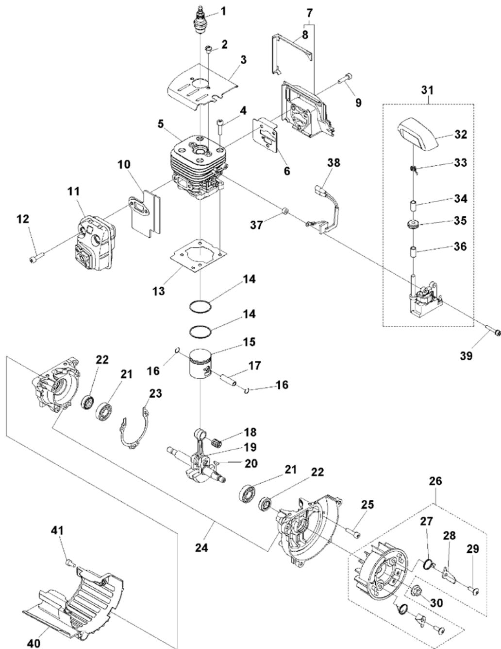
図1-エンジン
