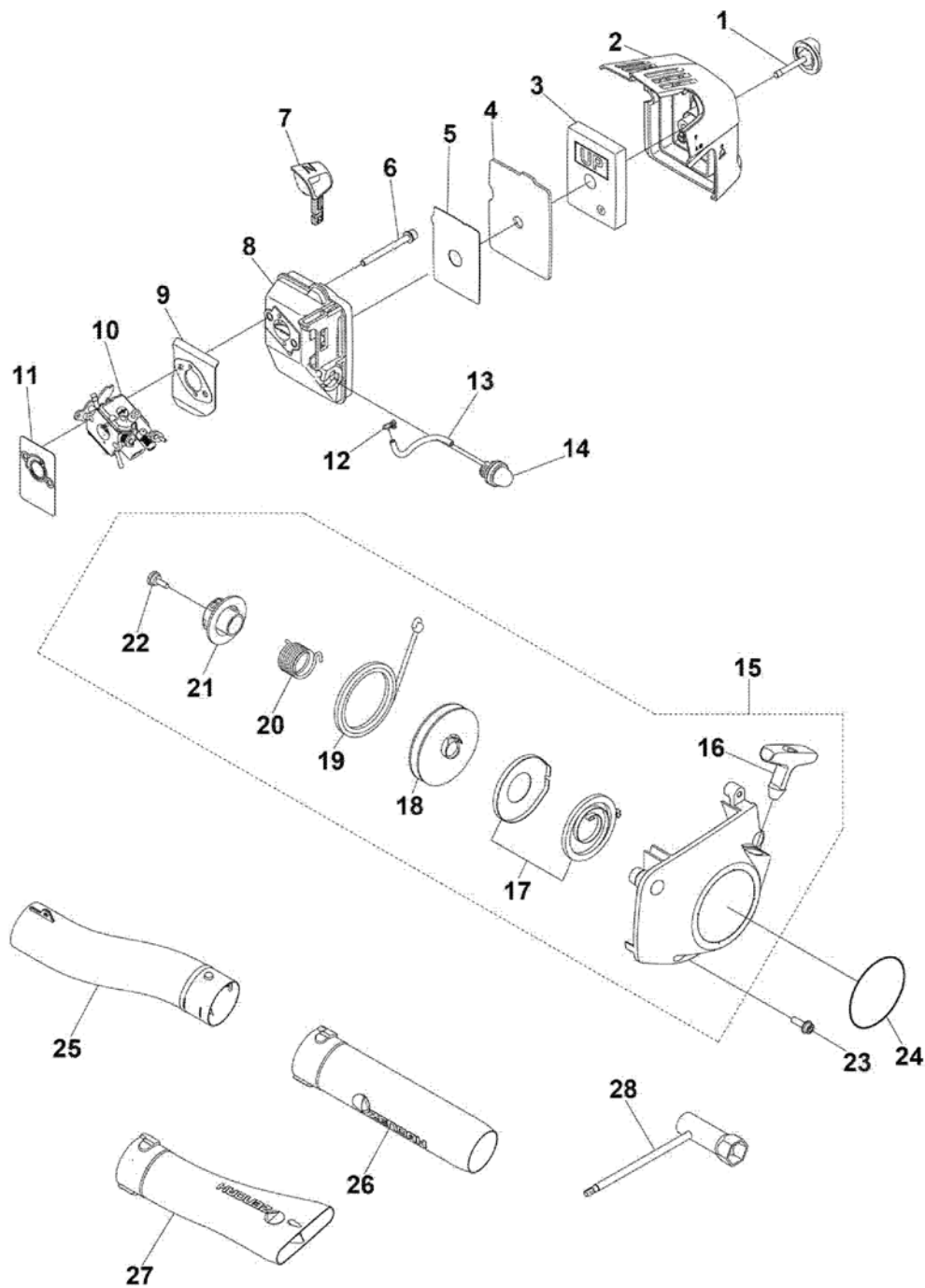
図3-吸気系・リコイル・付属品
