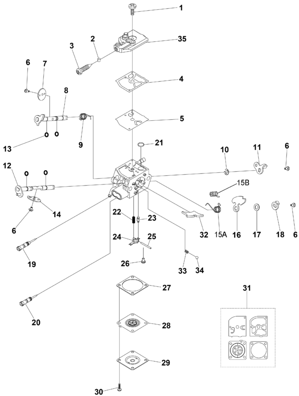
図-4 キャブレタ
